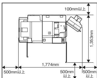
ステイブルフィニッシャー・V2装着時
