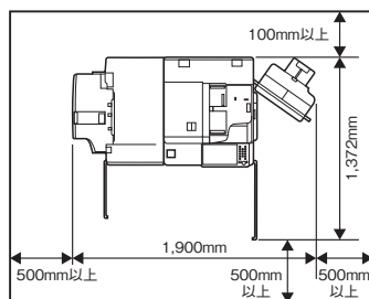
ステイブルフィニッシャー・X1装着時
