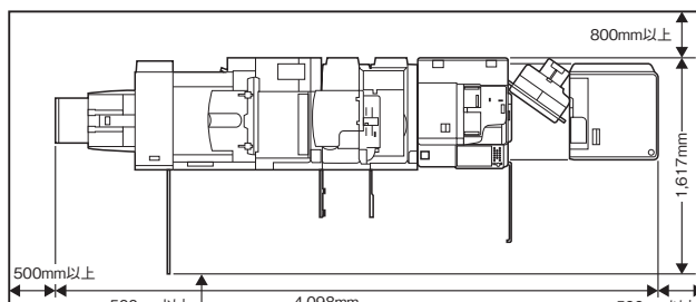
トリマー・D1+中綴じフィニッシャー・W1+ ペーパーフォールディングユニット・J1+インサーター・N1+ PODデキライト・C1装着時
