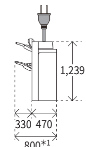
ステイプル フィニッシャー・AF1
