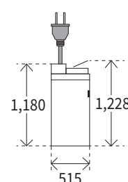
センシング ユニット・B1
