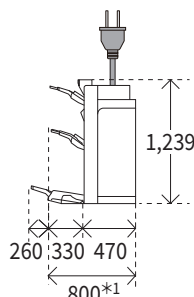
中綴じ フィニッシャー・AF1
