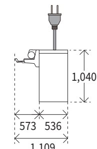
天地トリマー・B1 トリマーコンベア・B1
