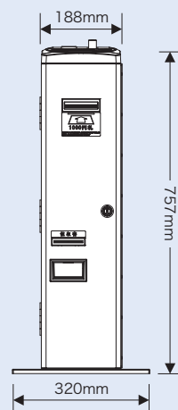
■ 占有スペース（正面図）
